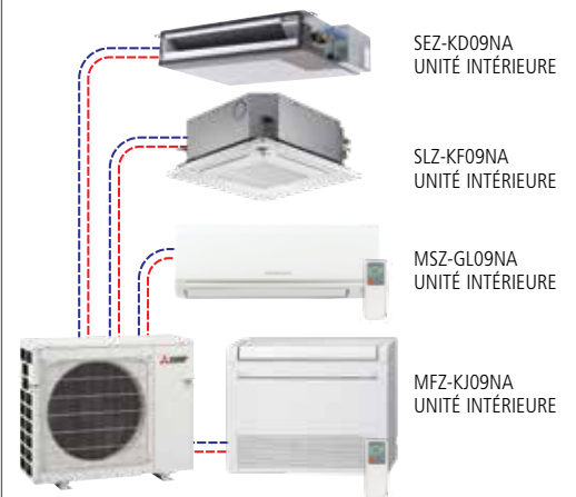
MXZ-4C36NA (2:1, 3:1, 4:1) UNITÉ EXTÉRIEURE
